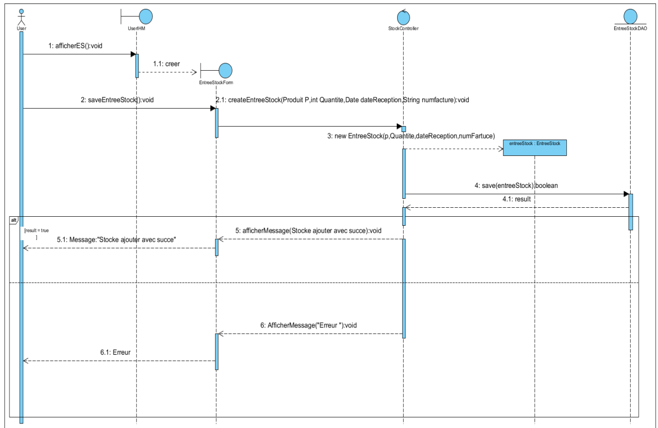
Figure 10 : Système d'interaction ajouter enrtee Stock
